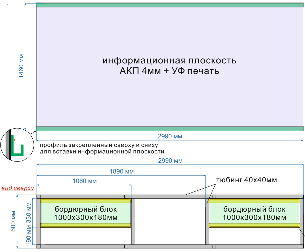
каркас сварной из тюбинга 40x40мм и уголка 50x50мм 3шт
