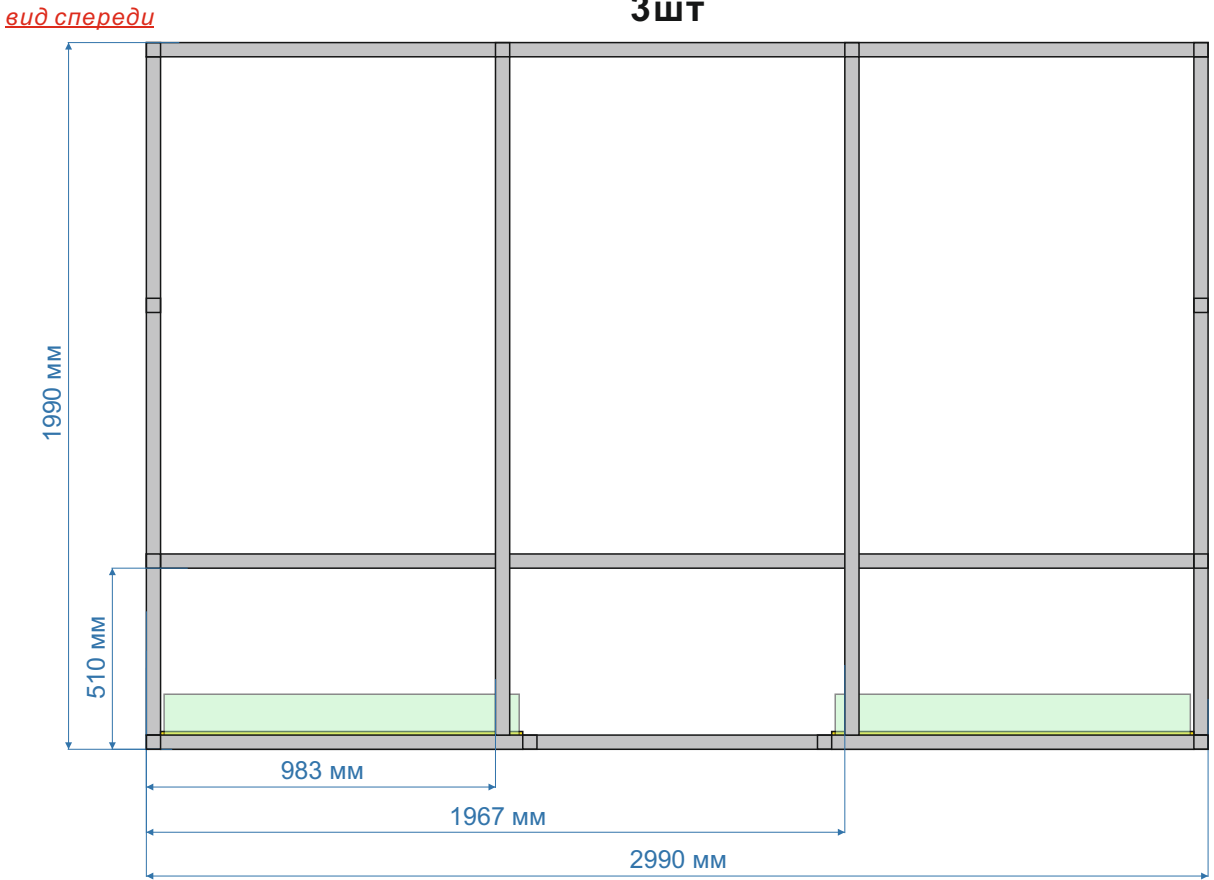
каркас сварной из тюбинга 40x40мм и уголка 50x50мм 3шт
