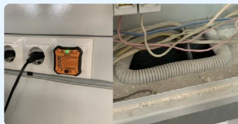
1. Розетки без заземления 2. Внутри щита пыль, грязь
