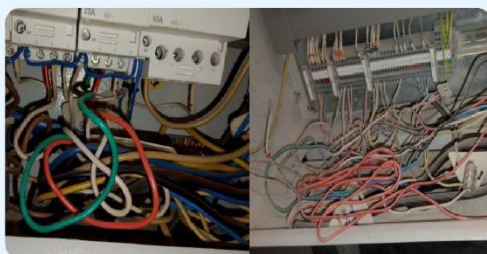
1. Монтаж кабеля неаккуратный, кабели не закреплены
