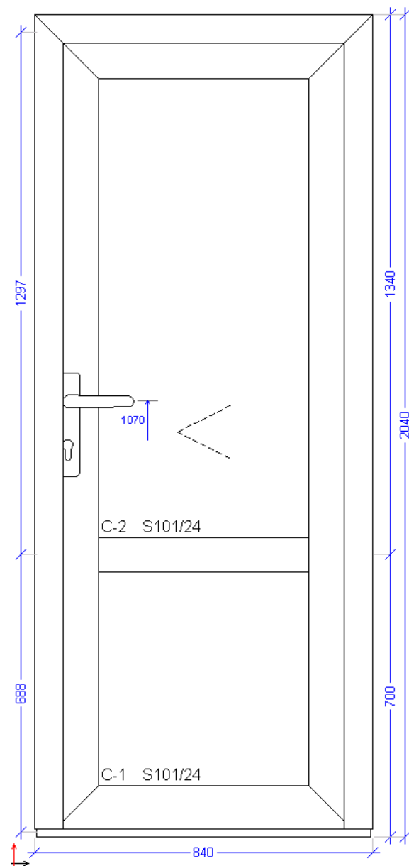
Схема Входная дверь ПВХ № 10-12
