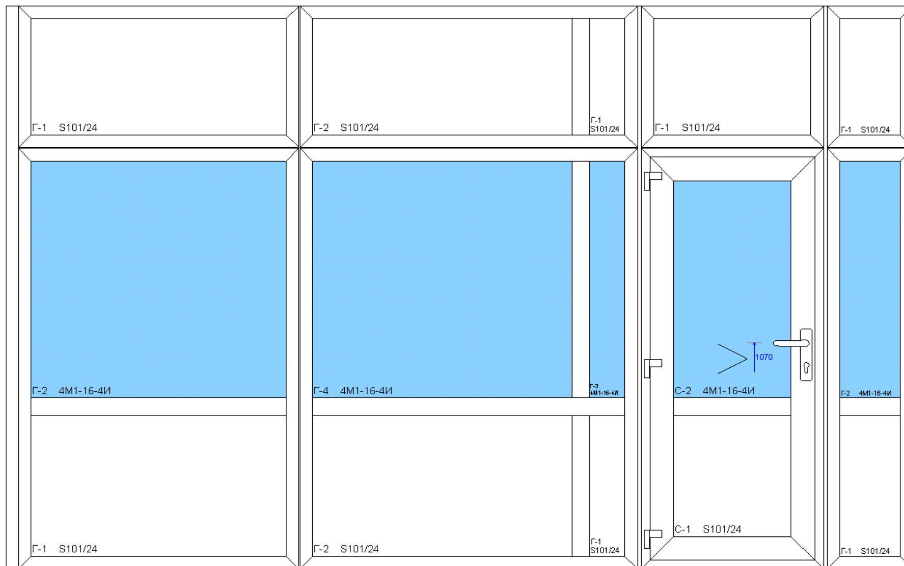
Схема Витраж с дверью № 1
