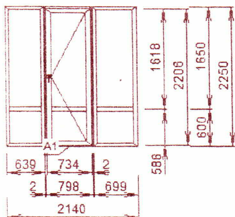
Изделие № 2 (Дверь входная в переход)
